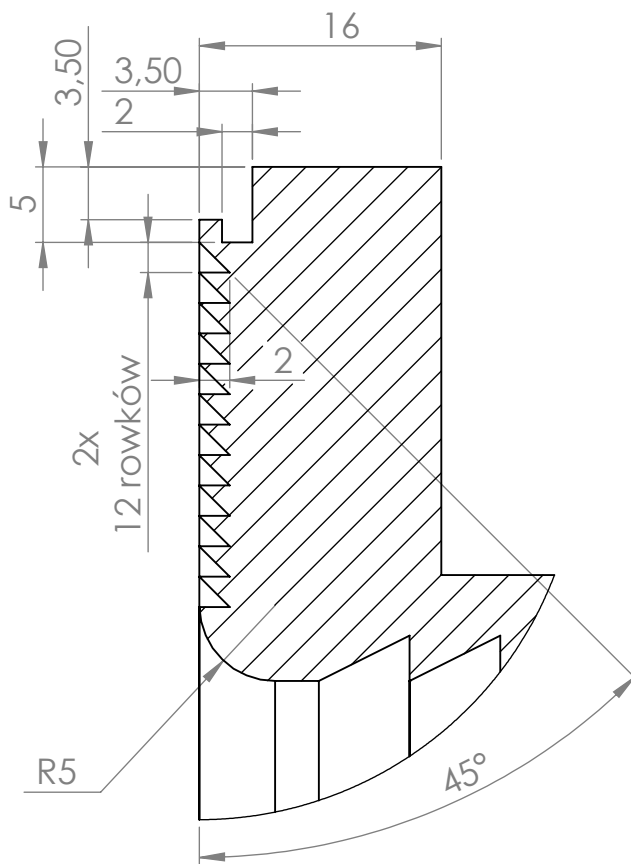
SZCZEGÓŁ B SKALA 2 : 1
